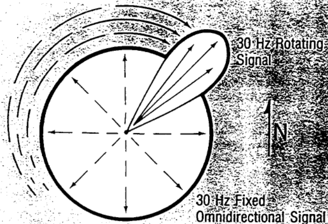
VOR Antenna Pattern
